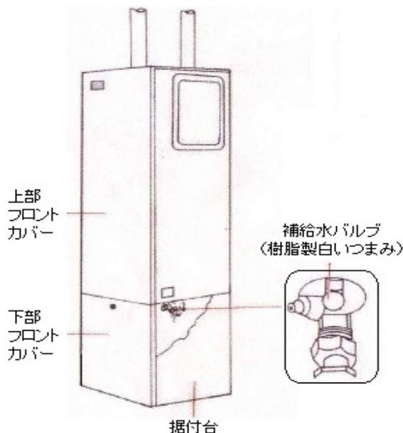
ガス給湯暖房機外観
