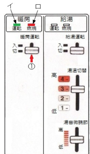
リモコンスイッチ
