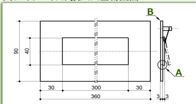
図3 ドアポスト投入口金物図面
