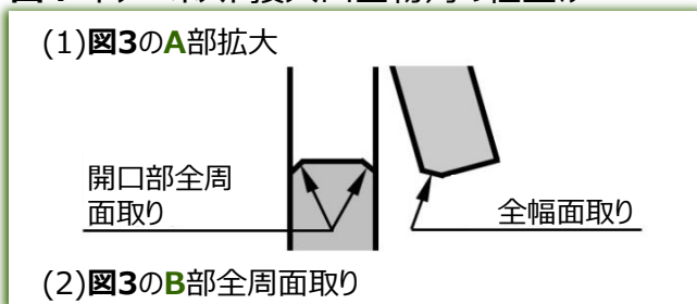
図4 ドアポスト投入口金物角の仕上げ
